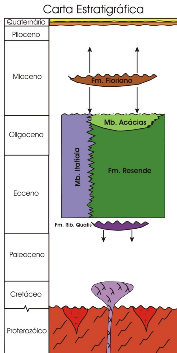
Figura 1. Carta estratigráfica da Bacia de Resende. Fonte: Ramos et al. (2006)
